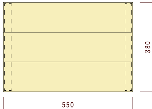
平面図（上から見た図）
