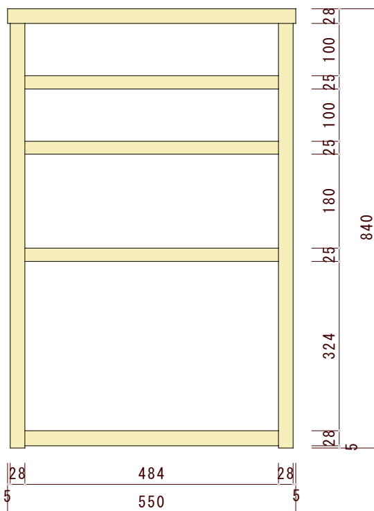
正面図（正面から見た図）
