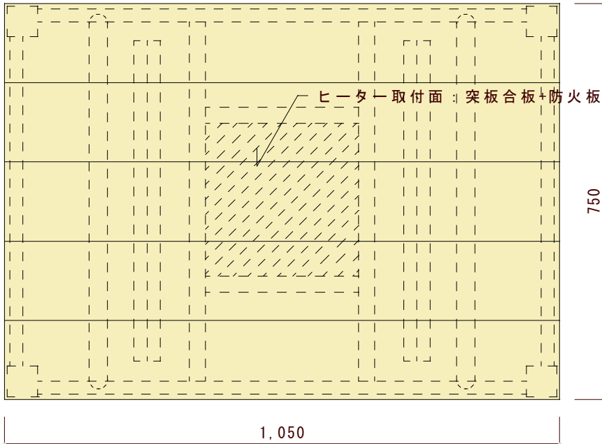
平面図（上から見た図）
