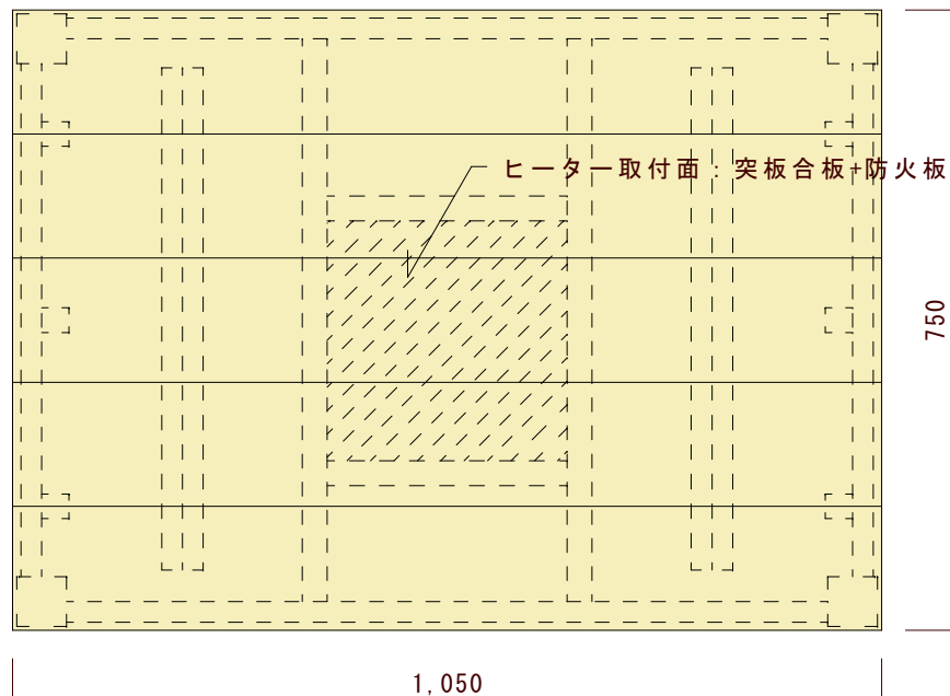
平面図（上から見た図）
