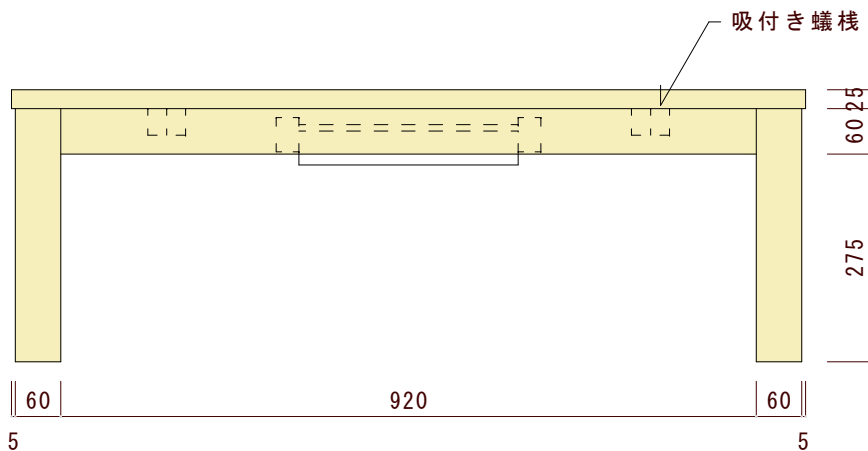
正面図（正面から見た図）
