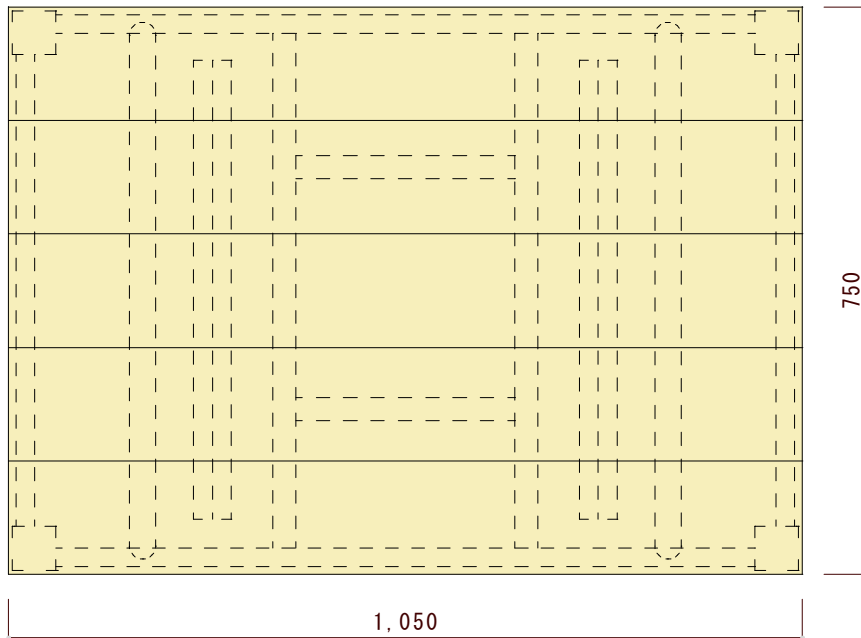
平面図（上から見た図）
