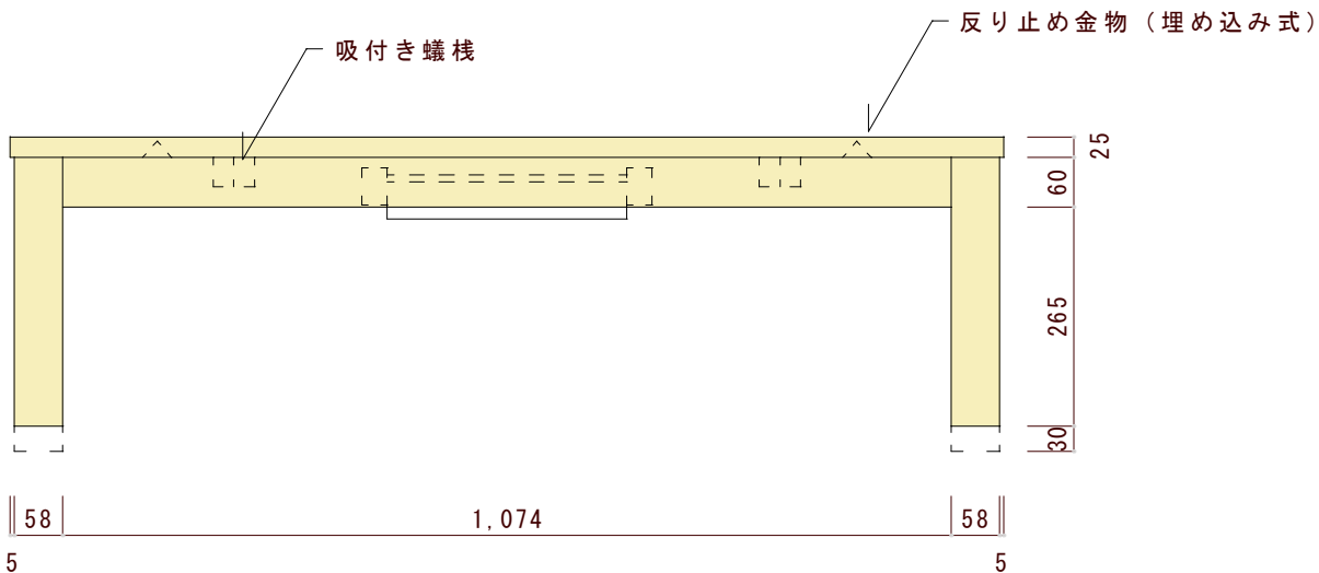
正面図（正面から見た図）
