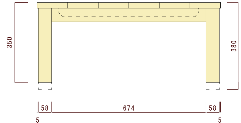
側面図（横から見た図）
