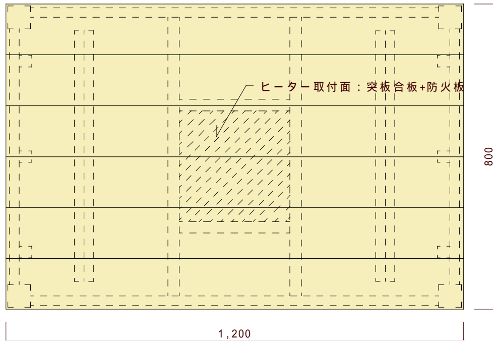
平面図（上から見た図）
