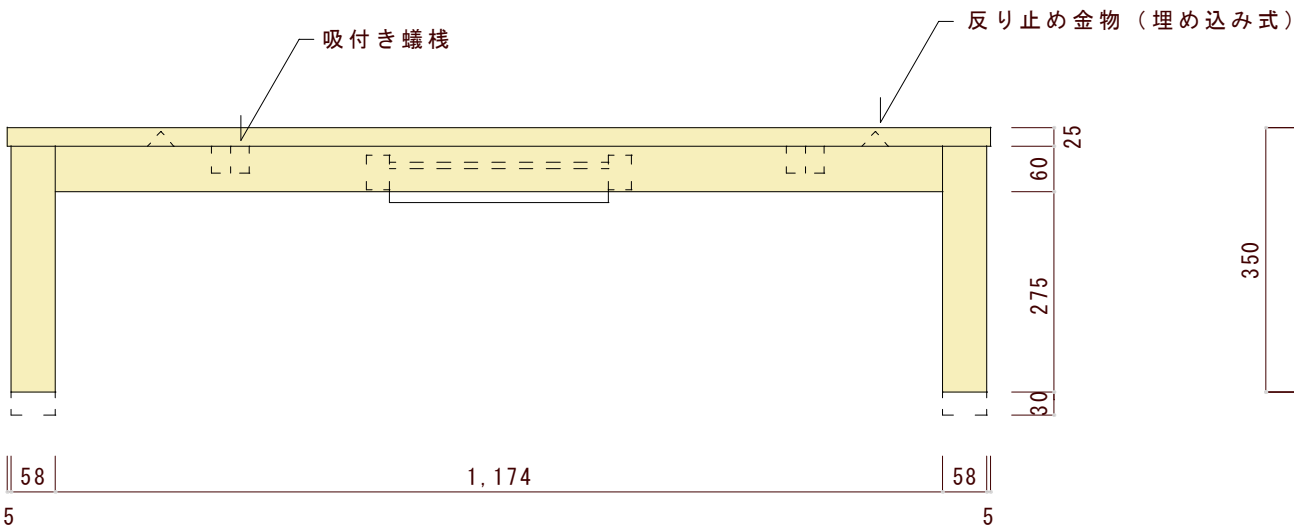
正面図（正面から見た図）
