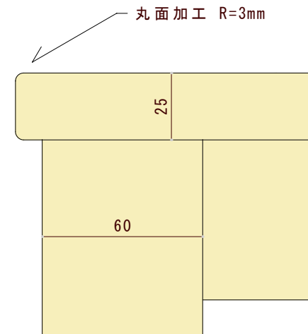
天板端部詳細図 S=1/2
