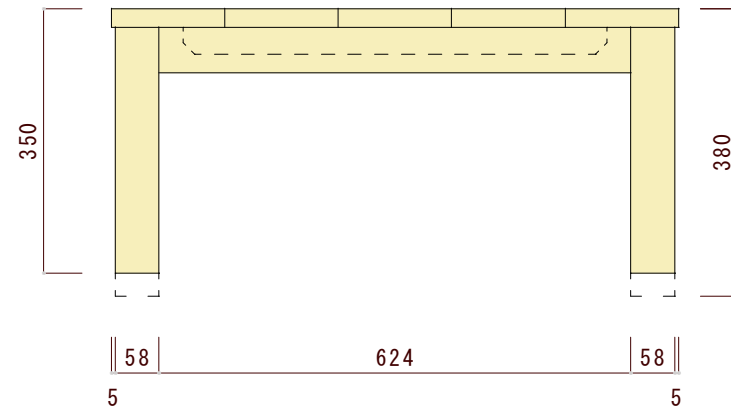
側面図（横から見た図）
