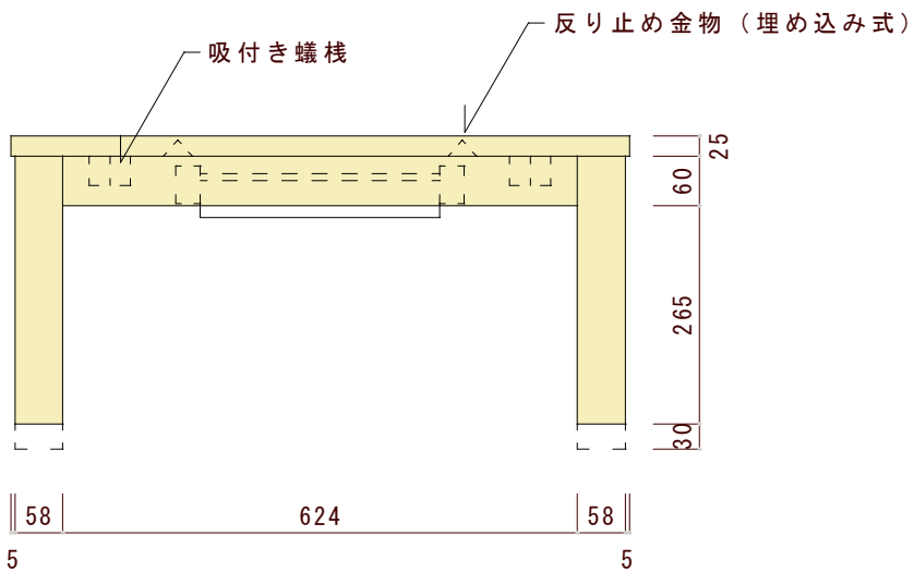
正面図（正面から見た図）
