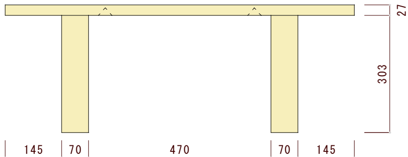
正面図（正面から見た図）
