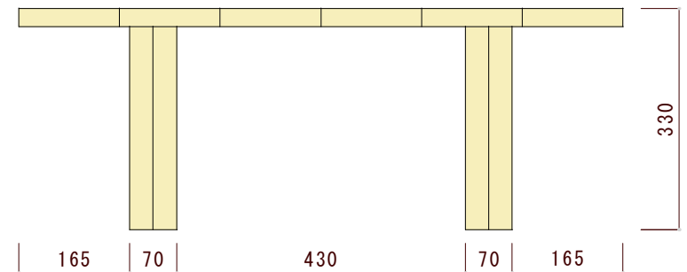
側面図（横から見た図）
