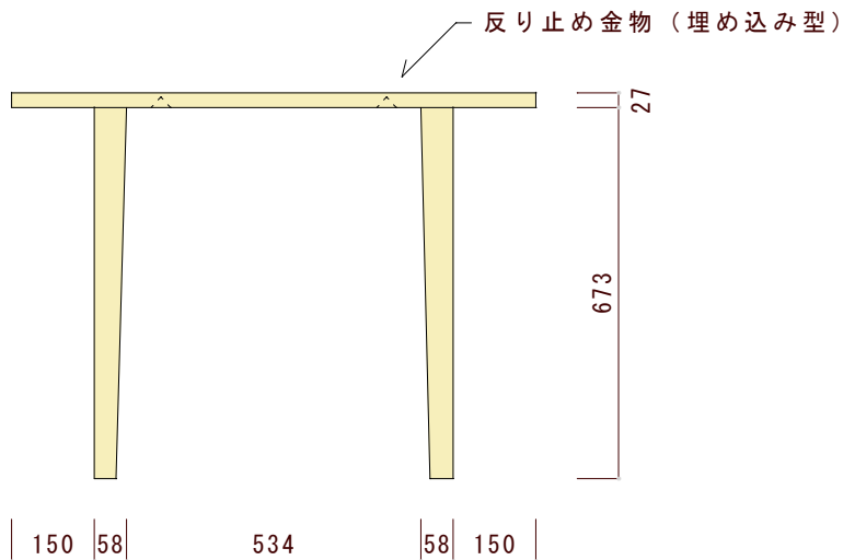
正面図（正面から見た図）
