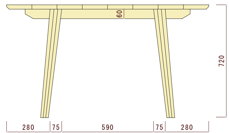
側面図（横から見た図）
