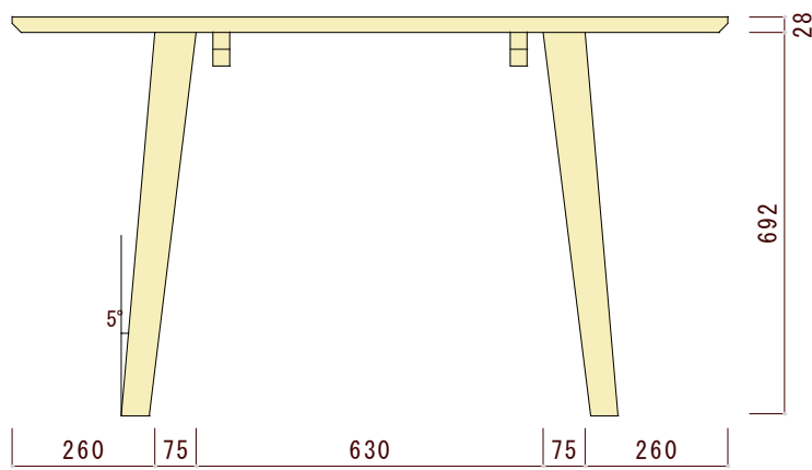
正面図（正面から見た図）
