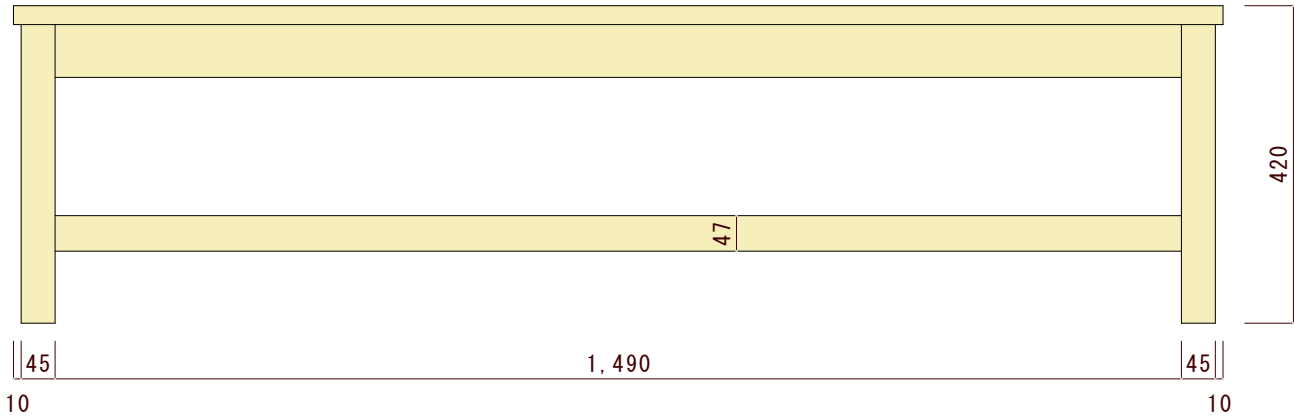
正面図（正面から見た図）
