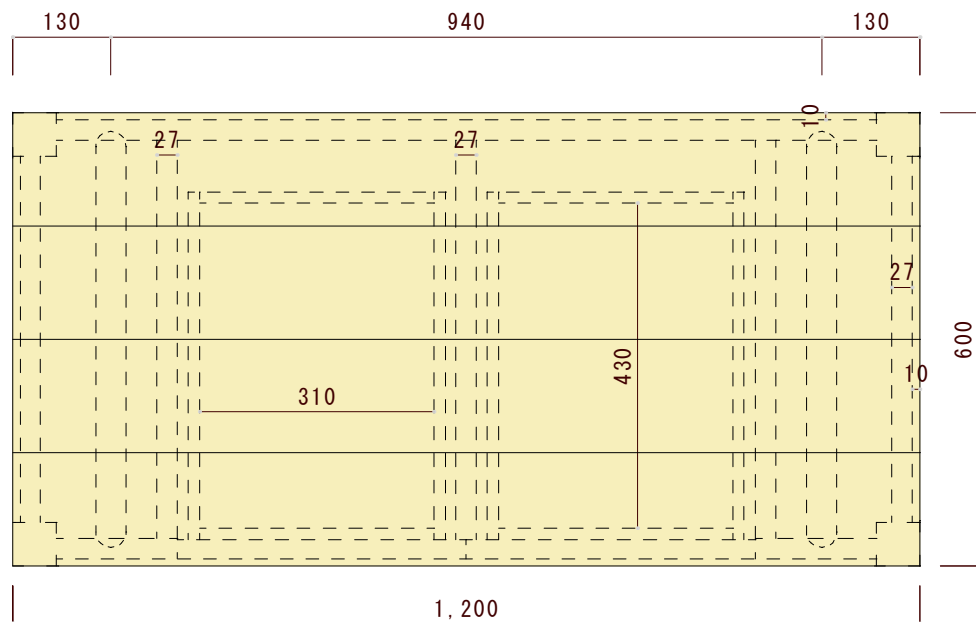
平面図（上から見た図）
