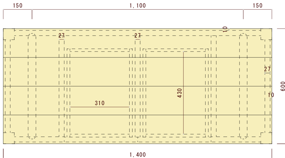
平面図（上から見た図）
