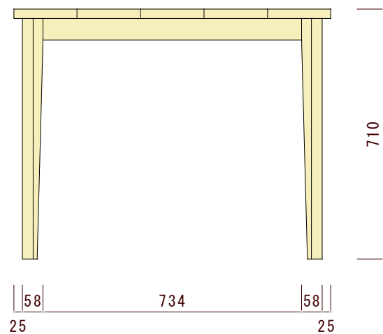
側面図（横から見た図）
