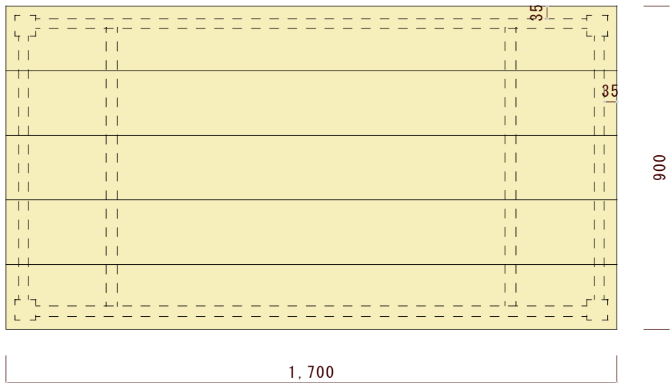
平面図（上から見た図）
