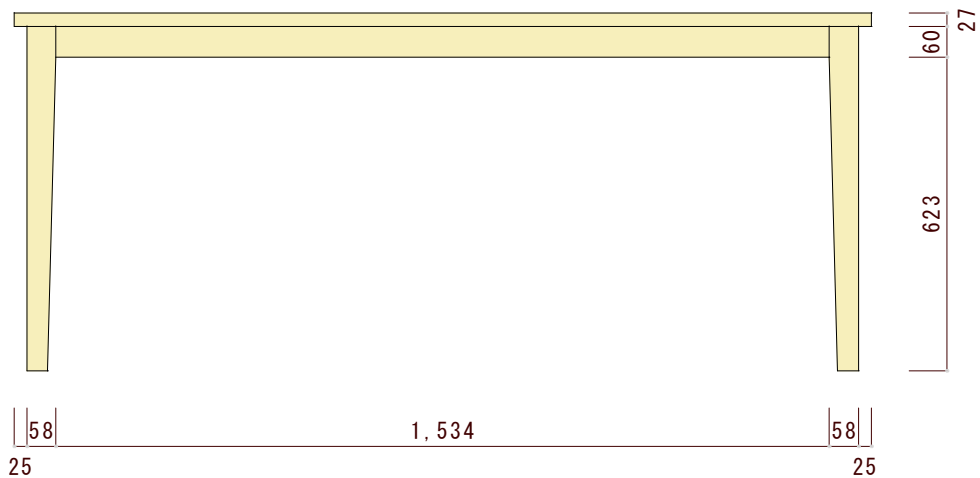
正面図（正面から見た図）
