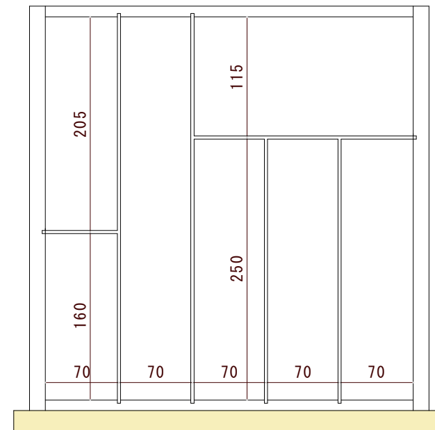
引出仕切り板配置図 S=1/5
