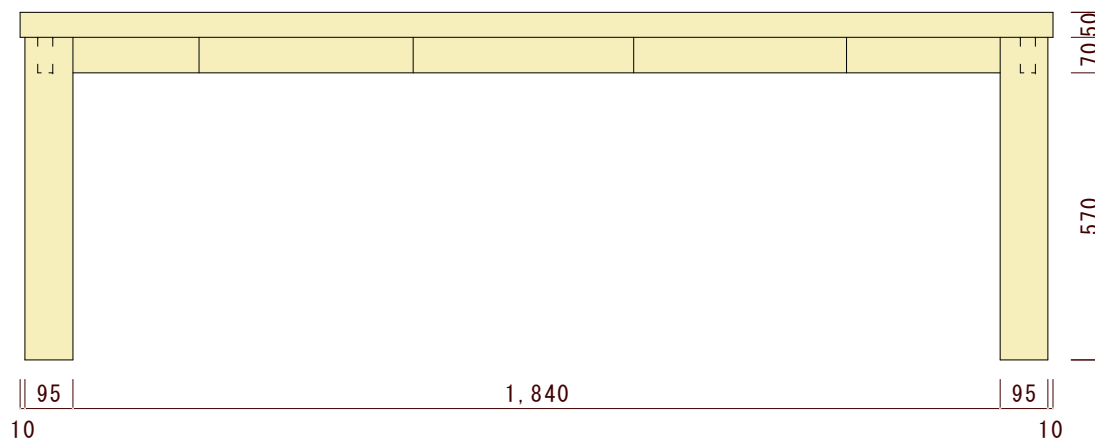
正面図（正面から見た図）
