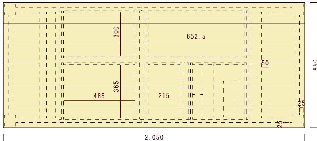
平面図（上から見た図）
