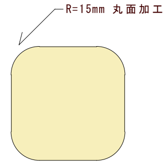
脚材断面図 S=1/2
