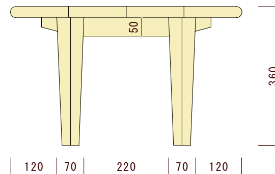
側面図（横から見た図）
