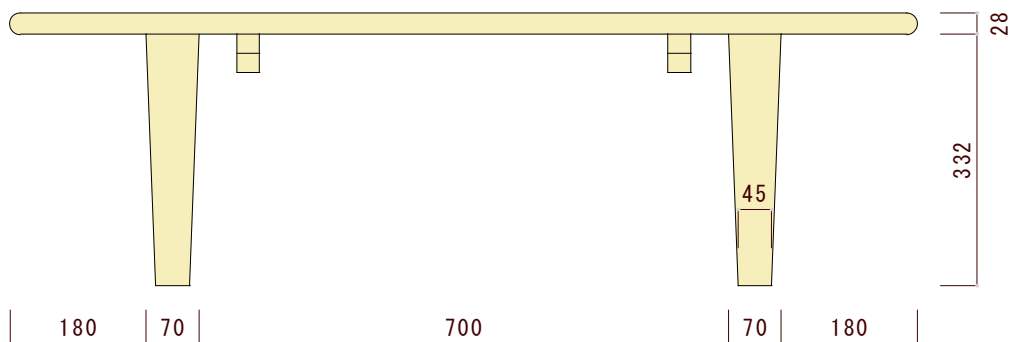
正面図（正面から見た図）
