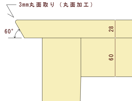
天板端部詳細図 S=1/3
