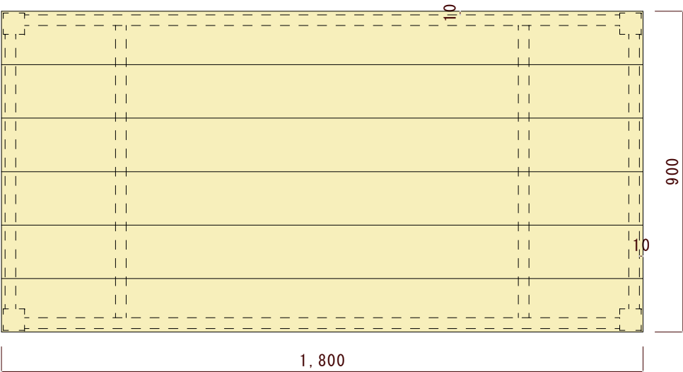
平面図（上から見た図）
