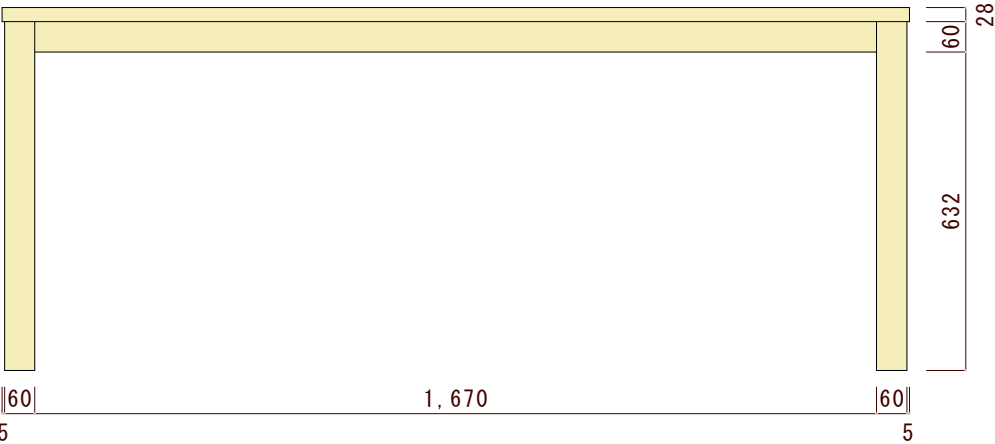
正面図（正面から見た図）
