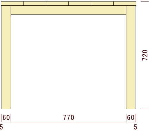
側面図（横から見た図）
