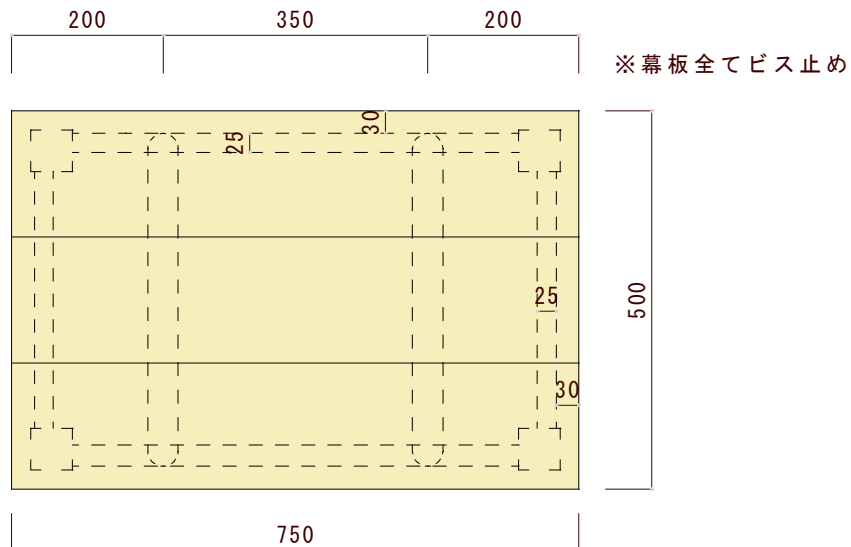
平面図（上から見た図）
