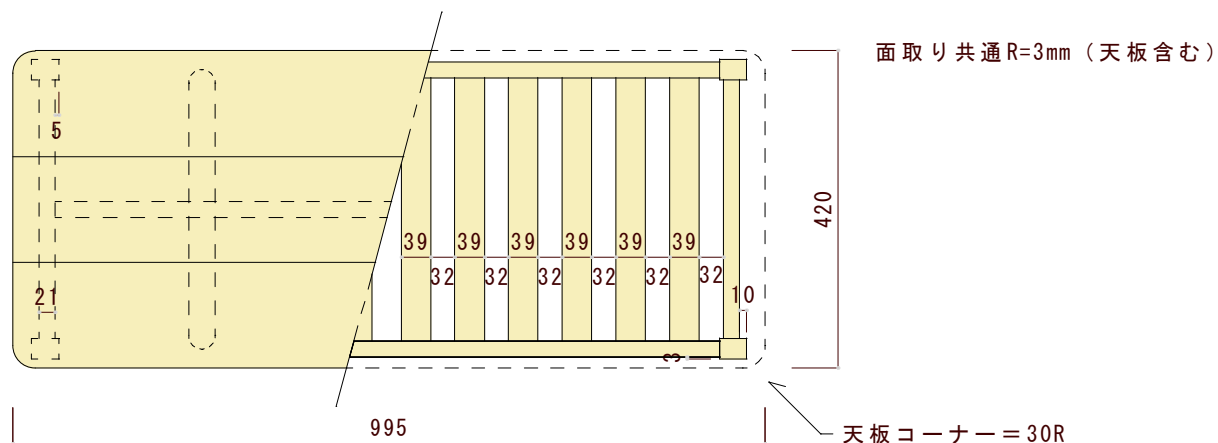
平面図（上から見た図）
