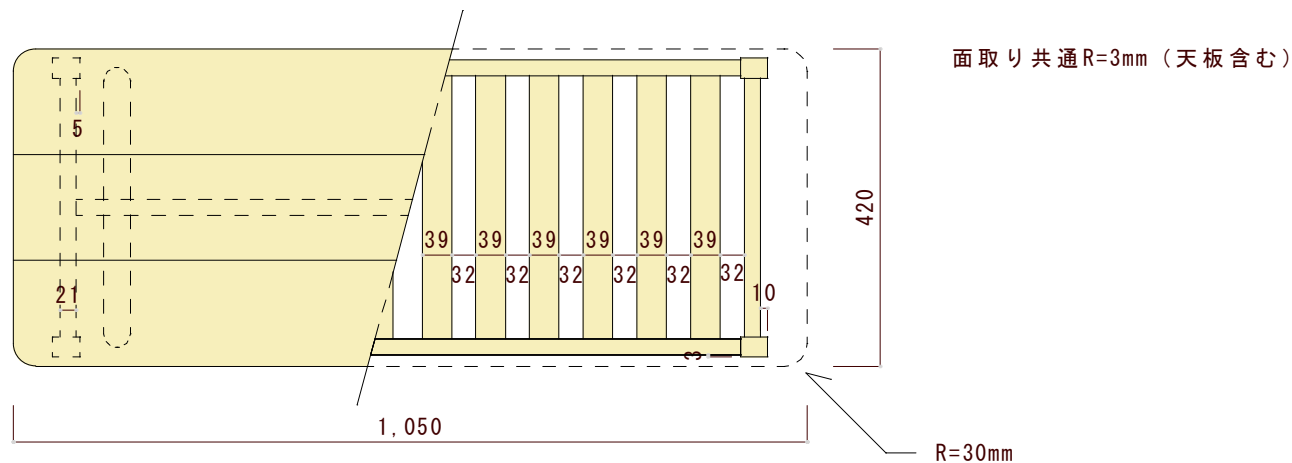
平面図 (上から見た図)
