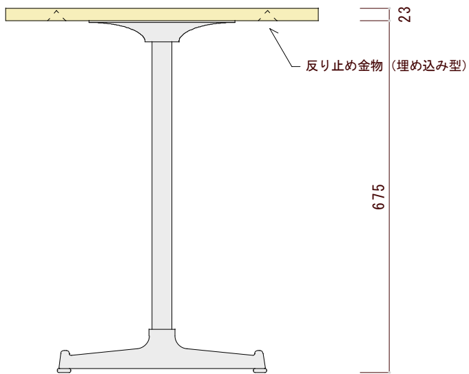
正面図（前から見た図）
