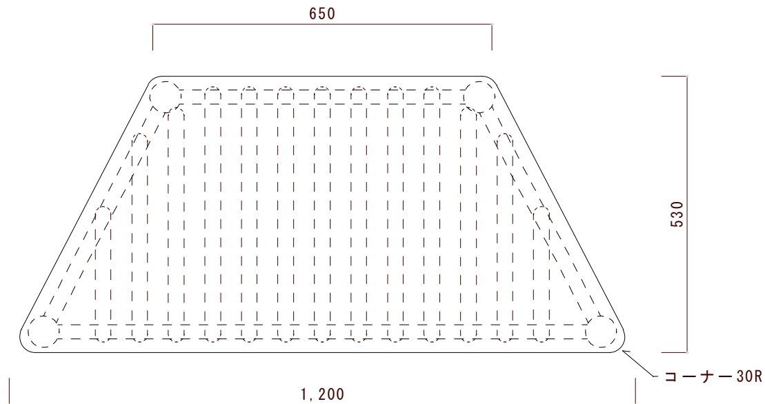
平面図（上から見た図）
