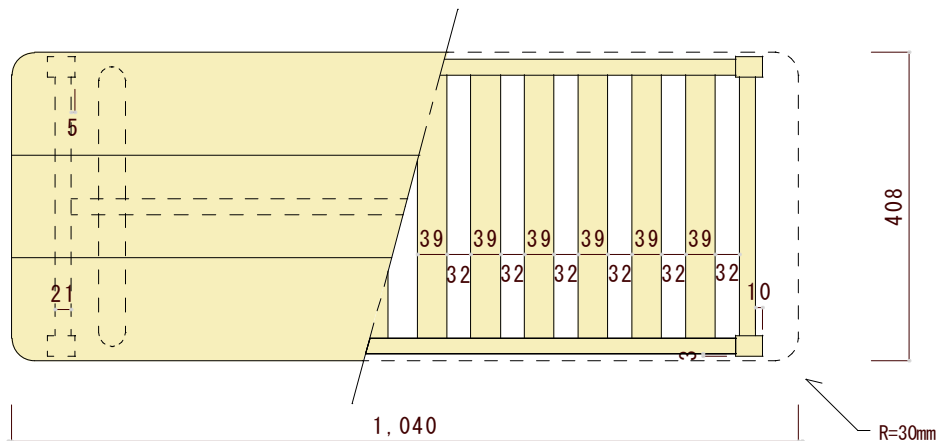
平面図（上から見た図）
