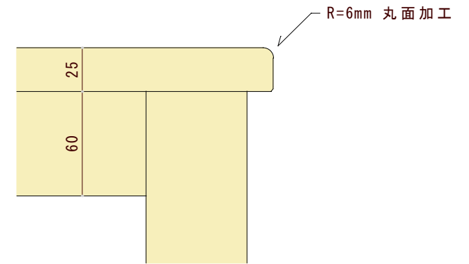
天板端部詳細図 S=1/3
