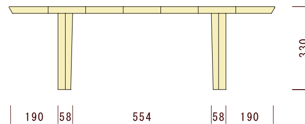
側面図 (横から見た図)
