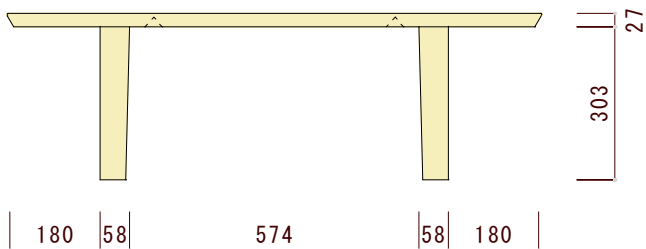
正面図 (前から見た図)
