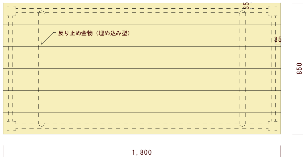
平面図（上から見た図）
