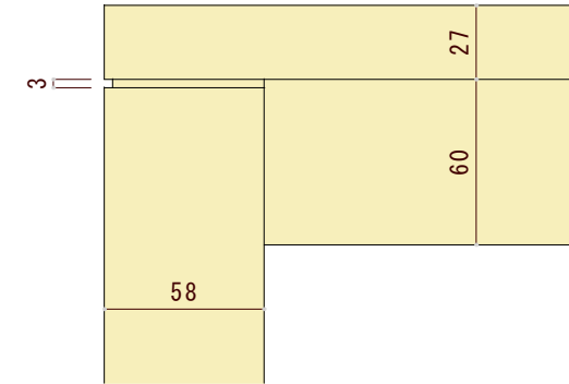
天板端部詳細図 S=1/3
