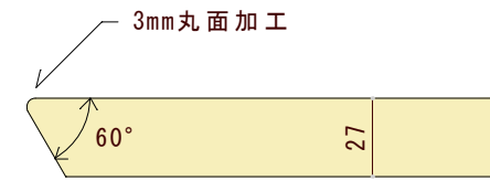
天板詳細図 S=1/3
