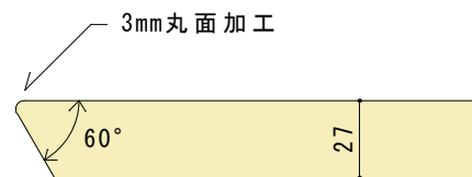
天板詳細図 S=1/3
