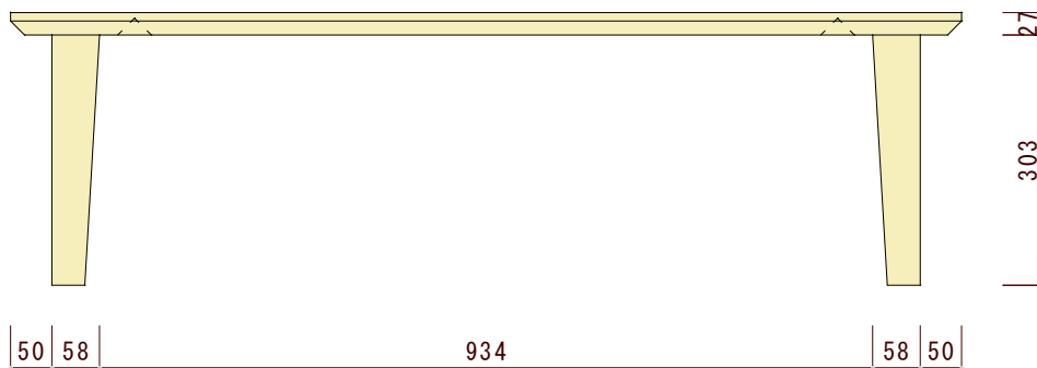
正面図 (前から見た図)
