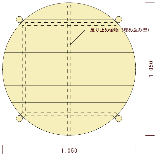
平面図（上から見た図）
